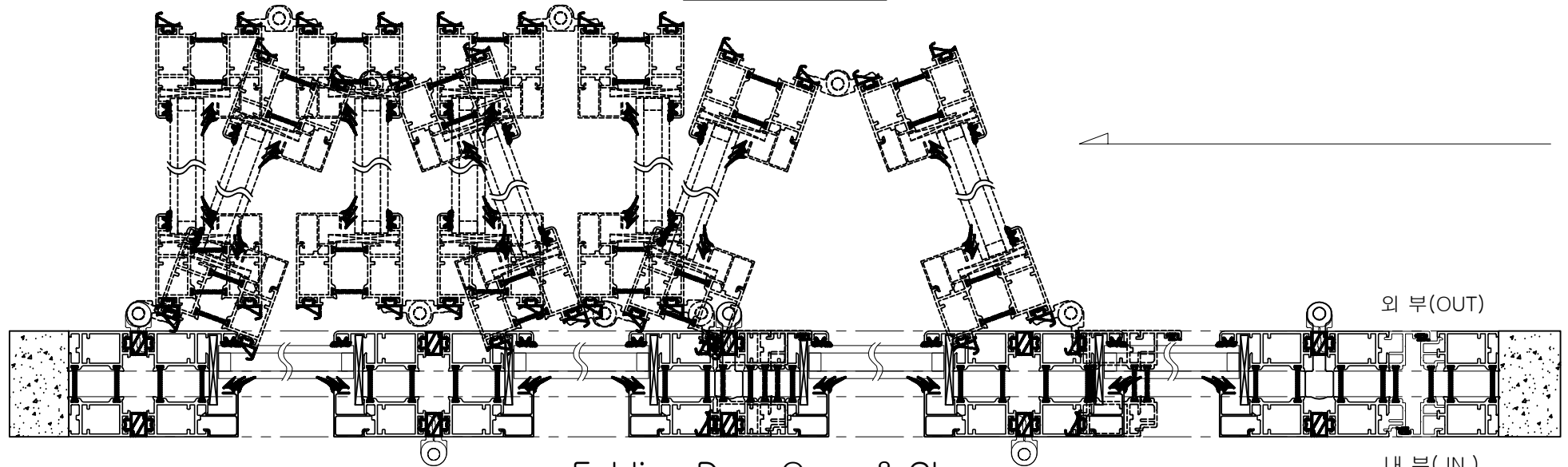
Folding Door Open & Close
