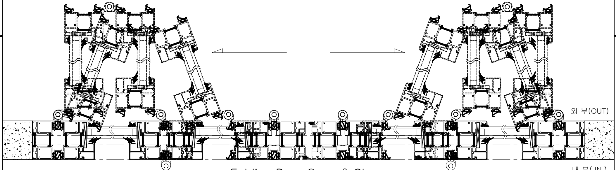
Folding Door Open & Close
