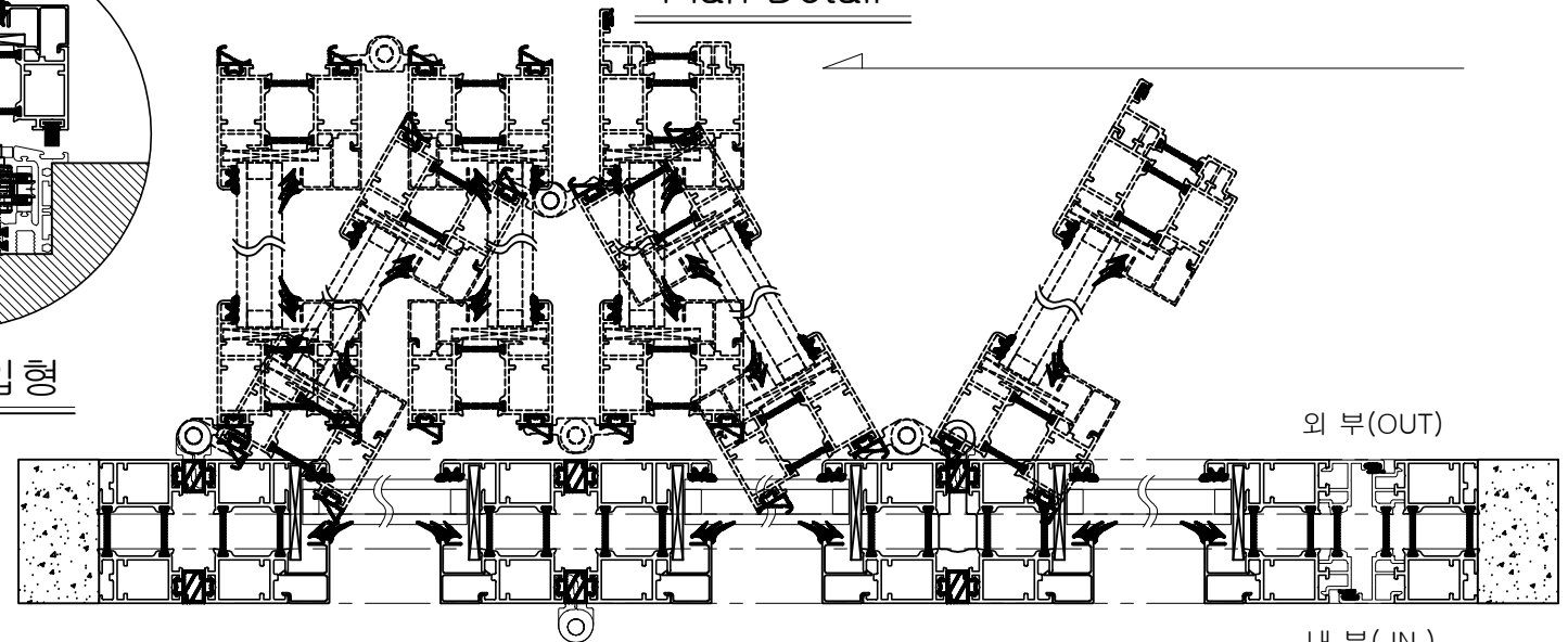
Folding Door Open & Close
